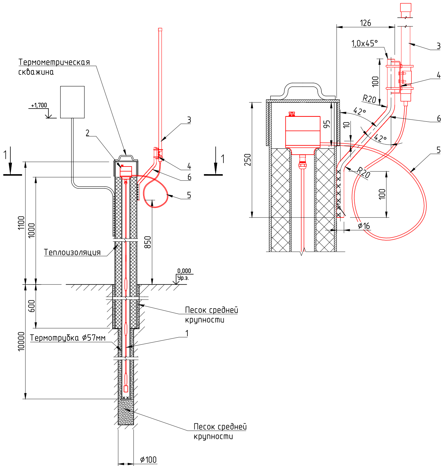
Общий вид крепления антенны
