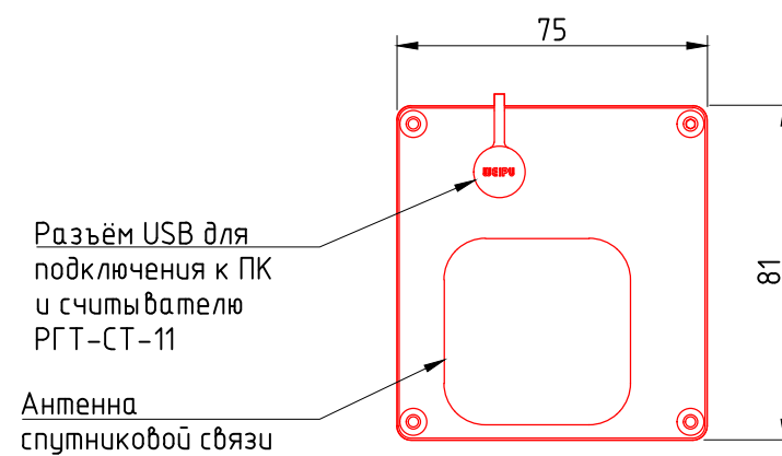
Вид сверху
