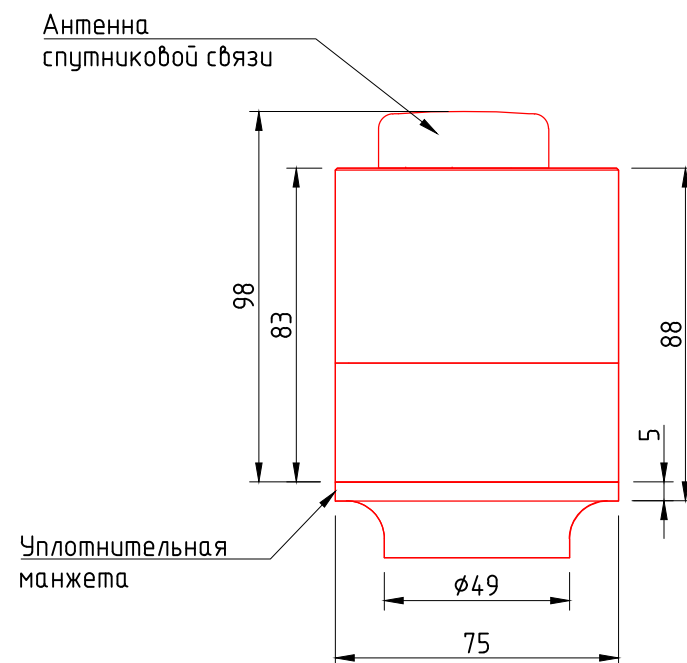
Вид спереди
