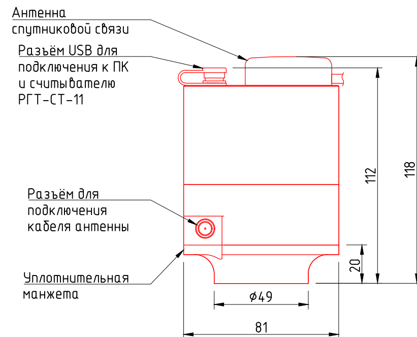
Вид сбоку
