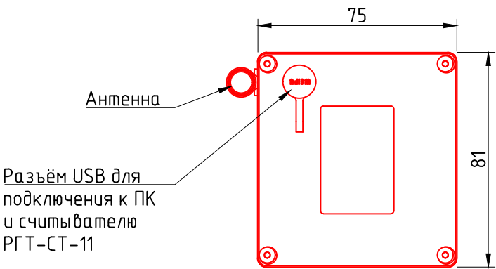
Вид сверху
