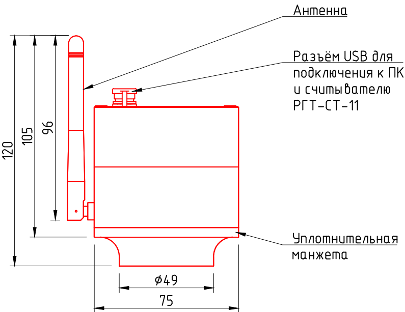
Вид спереди
