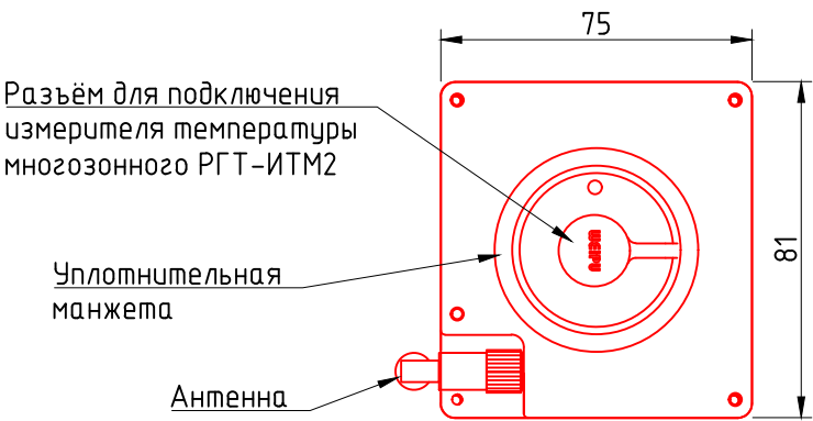
Вид снизу
