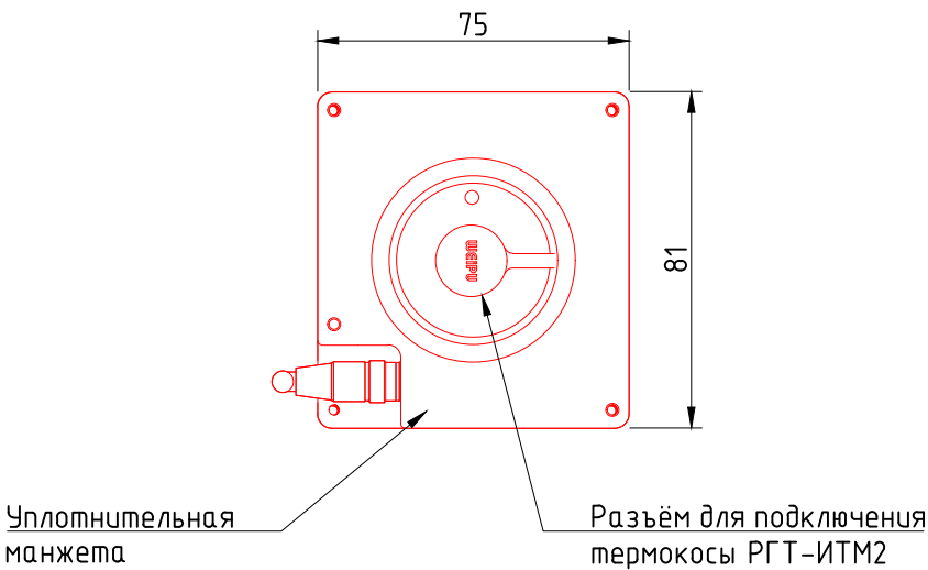
Вид снизу
