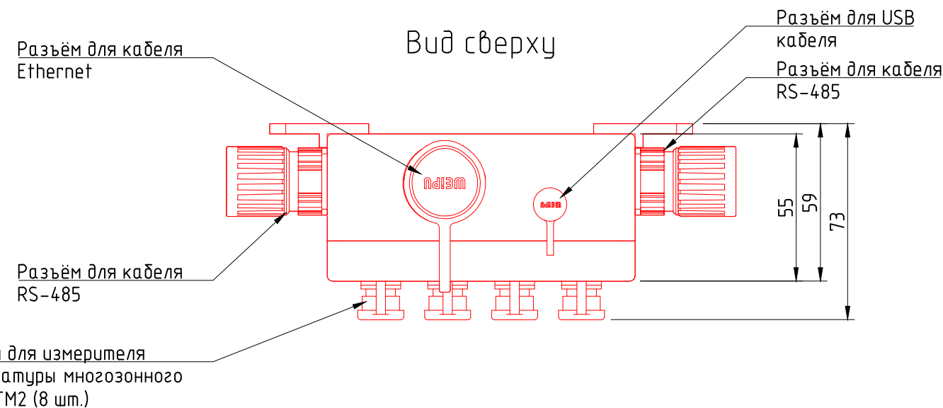
РГТ-КИТМ-10 с подключенными прямыми разъёмами кабеля RS-485
