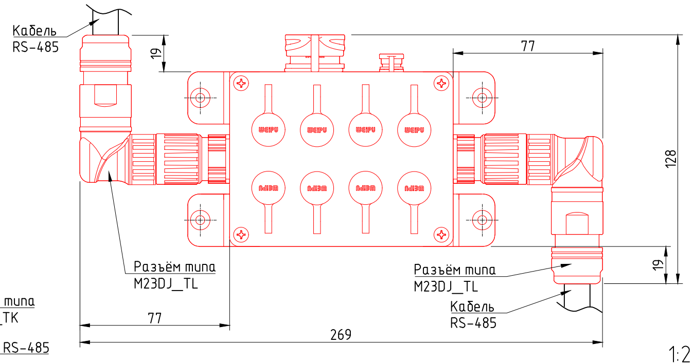
РГТ-КИТМ-10 с подключенными угловыми разъёмами кабеля RS-485
