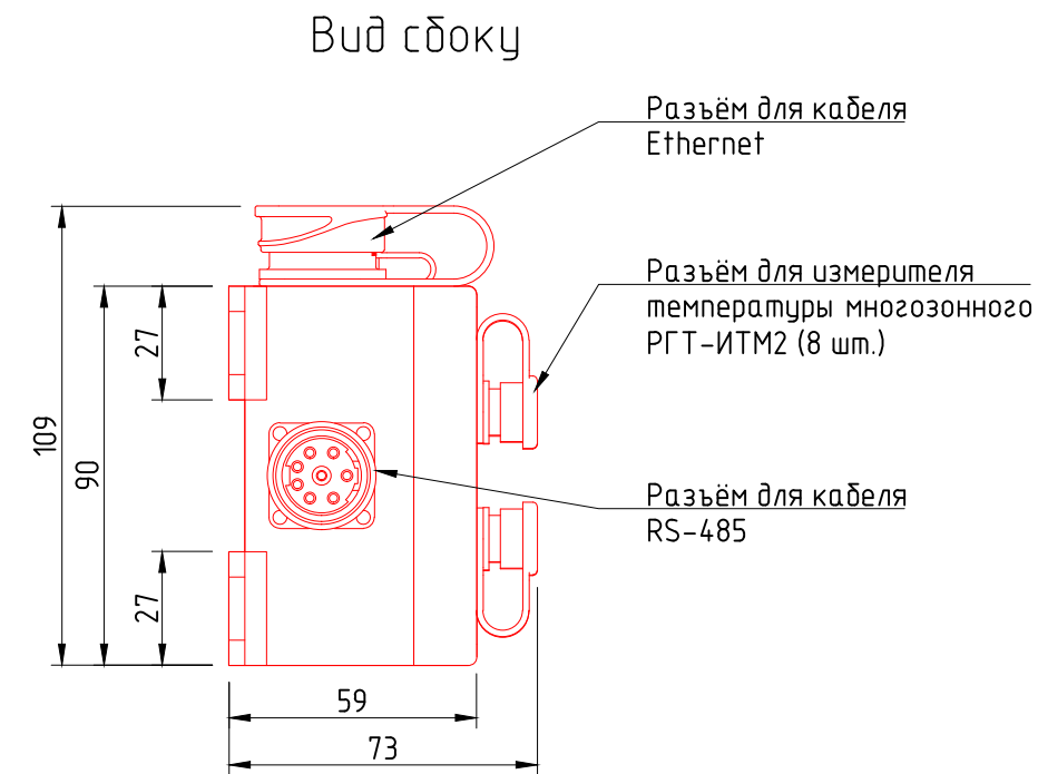
РГТ-КИТМ-10 с подключенными угловыми разъёмами кабеля RS-485
