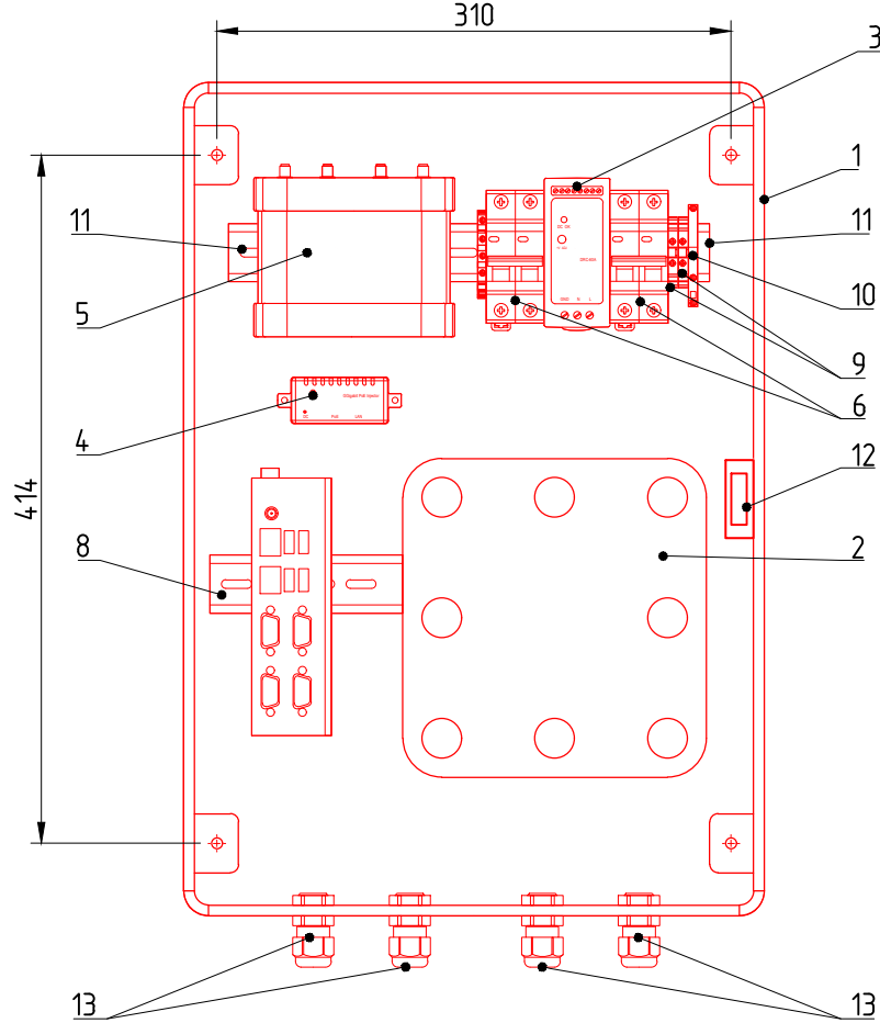
Комплектация блока
