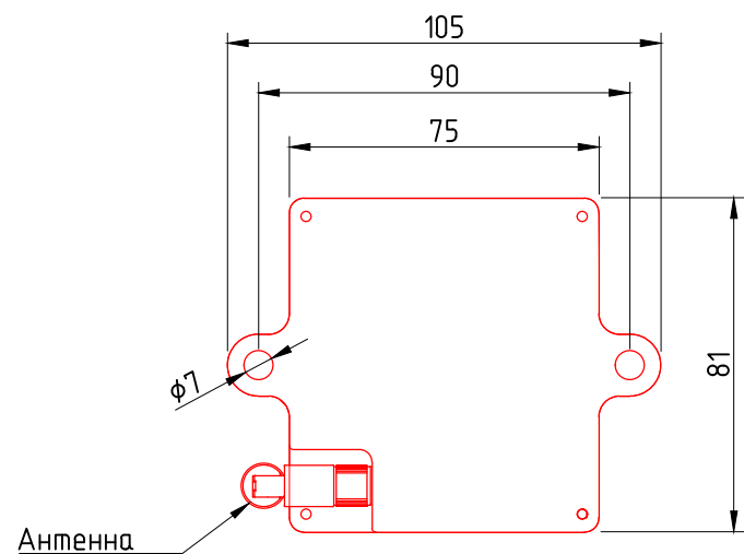
Вид снизу
