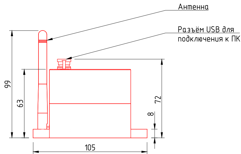
Вид спереди
