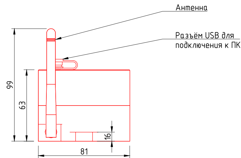
Вид сбоку
