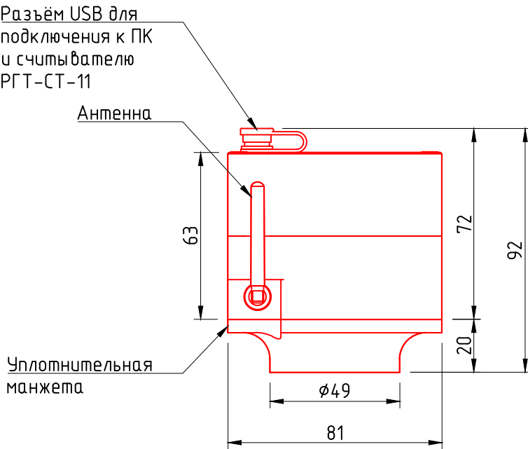
Вид сбоку
