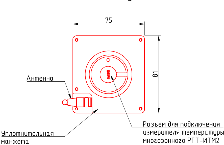
Вид снизу
