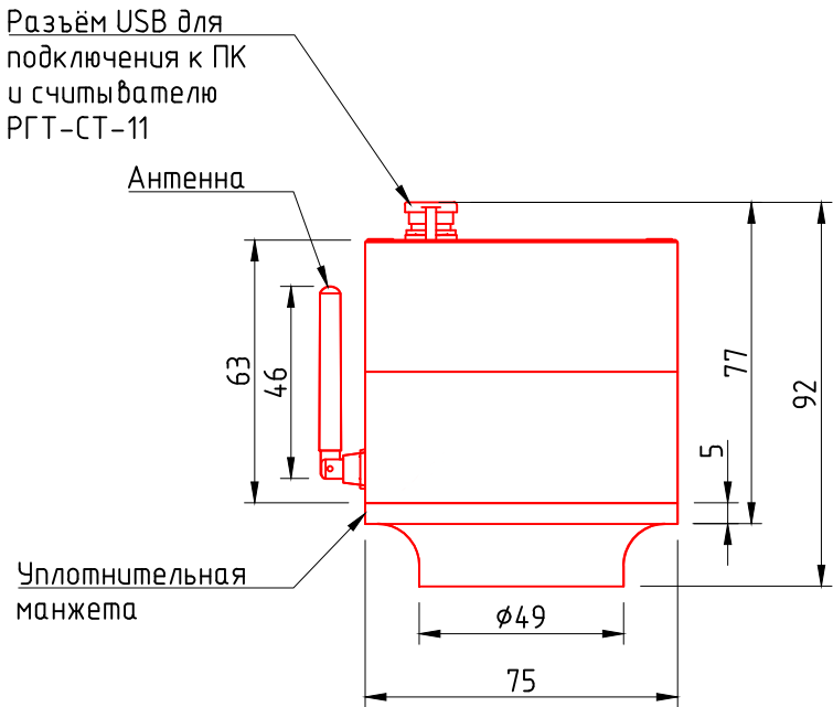
Вид спереди
