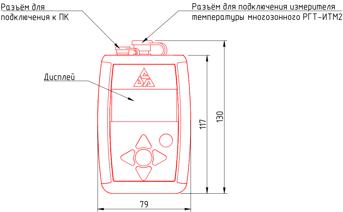
Вид спереди
