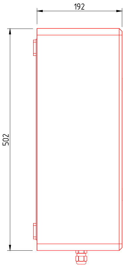
Вид сбоку
