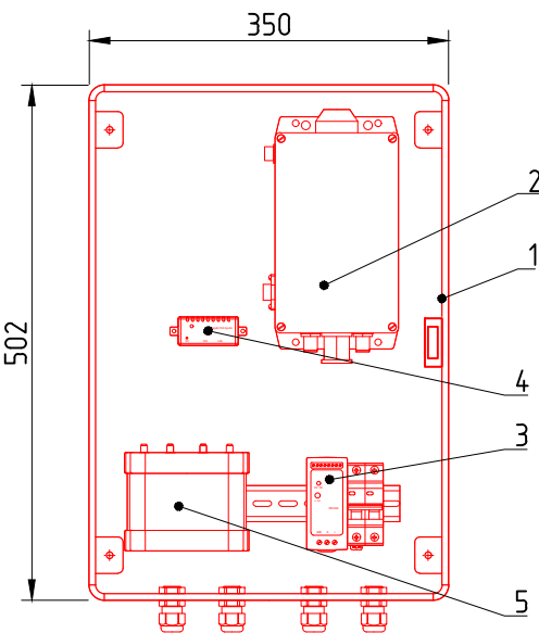
Блок выносной с БС
