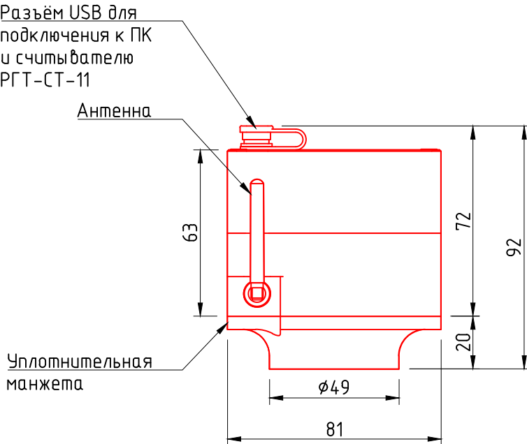
Вид сбоку
