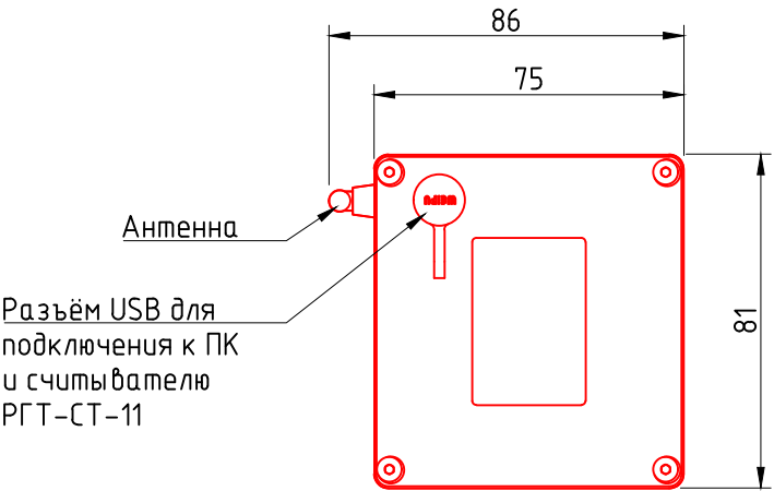
Вид сверху
