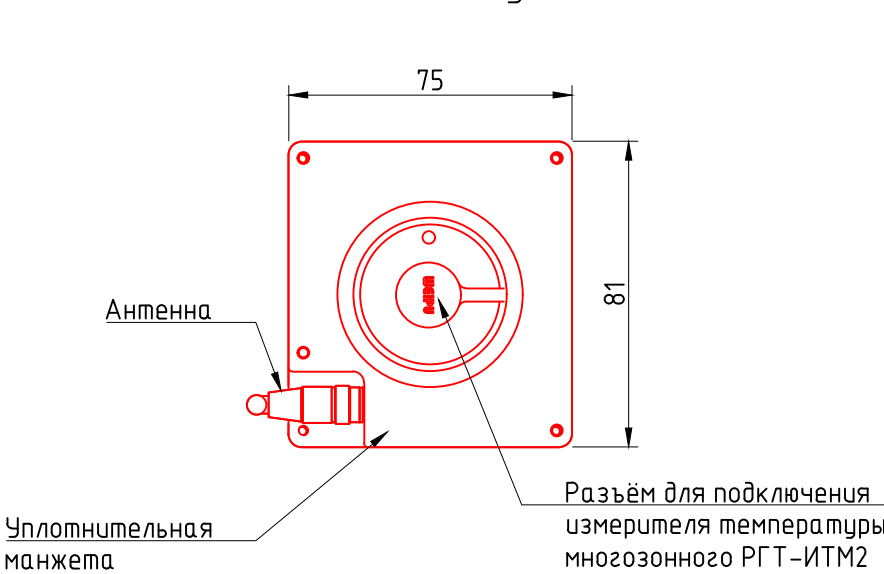
Вид снизу
