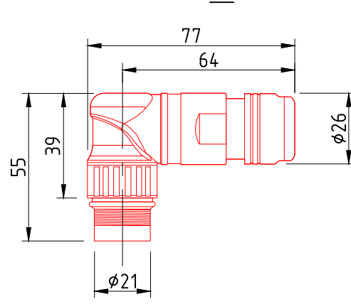
Разъём M23DJ_TL
