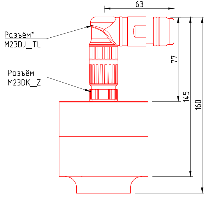
Вид сбоку с подключёнными разъёмами M23DJ_TL
