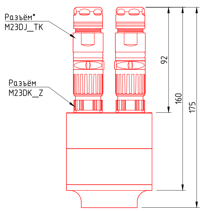
Вид спереди с подключёнными разъёмами M23DJ_TK
