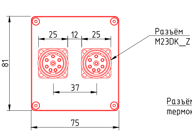
Вид сверху
