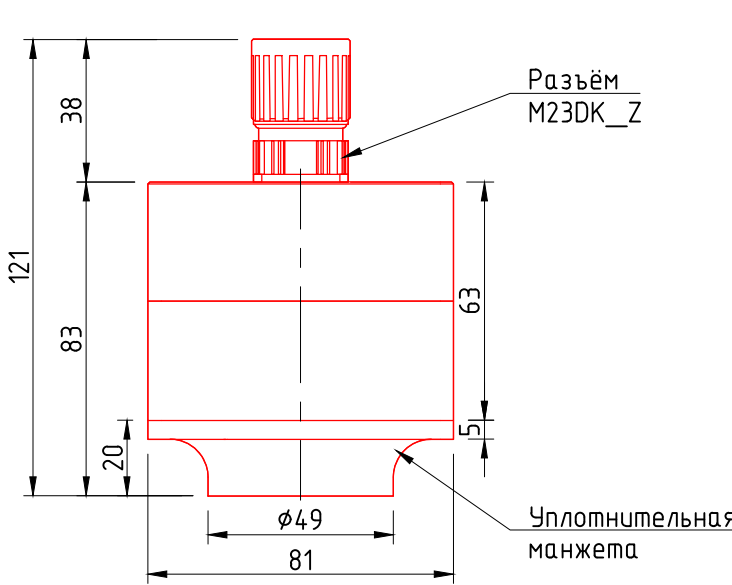
Вид сбоку
